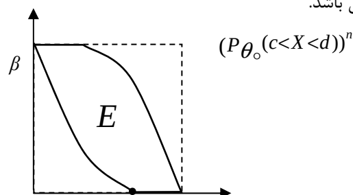
شکل ۱۰: مجموعه محدب نقاط خطی وقتی -\infty \leq a < c < d < b \leq +\infty
