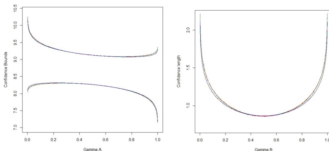
شکل ۲. حدود (A) و طول (B) فاصله اطمینان‌های حاصل از ۳ روش بر روی داده‌های موتور موشک
