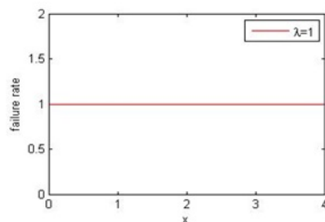
شکل ۵. نرخ شکست توزیع نمایی برای \lambda = 1 تابعی ثابت است.
