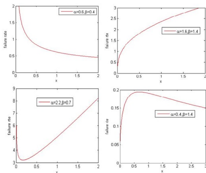
شکل ۸. نرخ شکست توزیع ENH برای مقادیر مختلف \alpha و \beta و \lambda = 1
