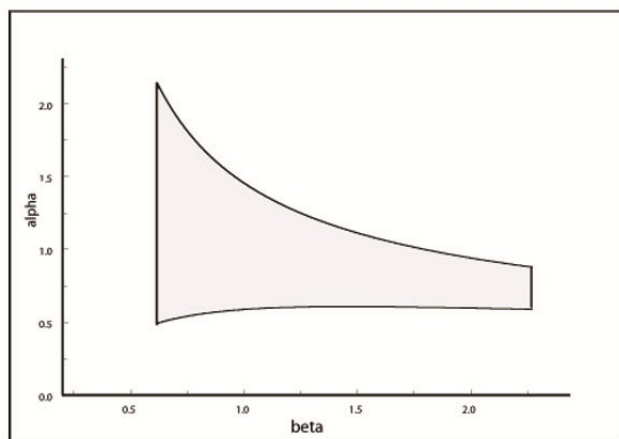
شکل ۴. ناحیه اطمینان دقیق در توزیع وایبل
