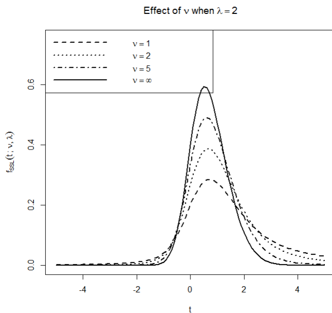
شکل ۲. نمودار تابع چگالی توزیع چوله-اسلش
