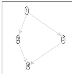
شکل ۴: دگ متشکل از ۴ متغیر دو وضعیتی W = 1, S = 2 ، R = 3 و C = 4 .
