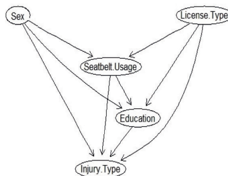
شکل ۸: ساختار به دست آمده با استفاده از الگوریتم PC
