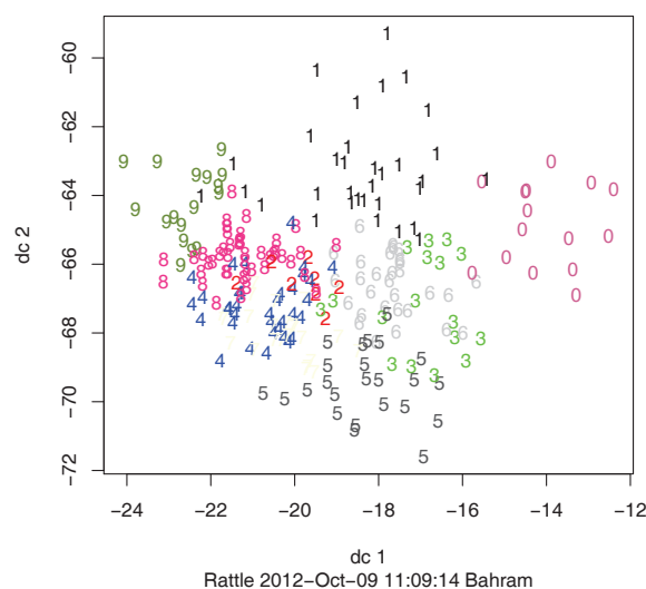
شکل ۷: نمودار تشخیصی برای مجموعه داده هواشناسی
