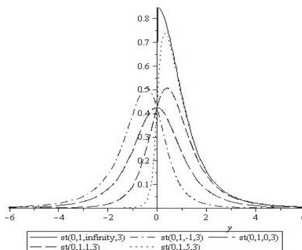
شکل ۱: تابع چگالی چوله-تی برای مقادیر مختلف \lambda
