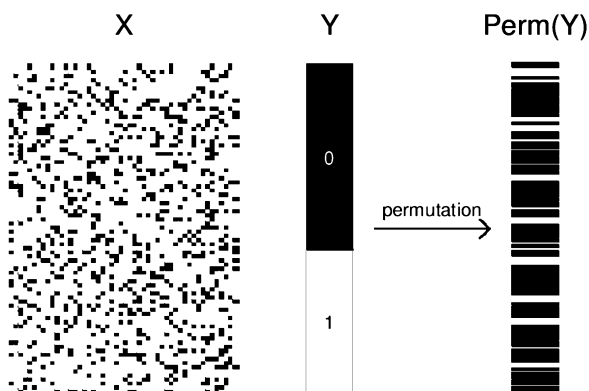
شکل ۳. آزمون تصادفی‌سازی
