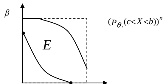
شکل ۹: مجموعه محدب نقاط خطا وقتی -\infty \leq a < c < b < d \leq +\infty
