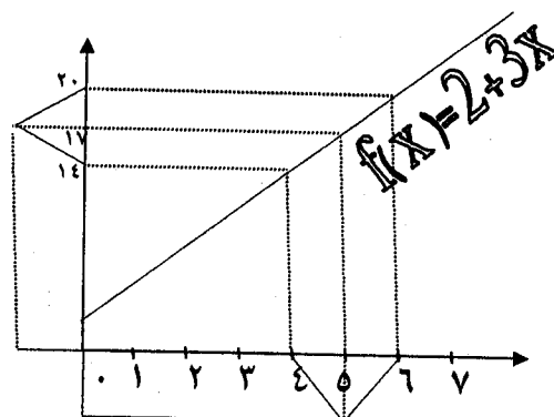
شکل ۳: محاسبه تخمین \tilde{y}_0 برای یک مقدار مشکک \tilde{x}_0
