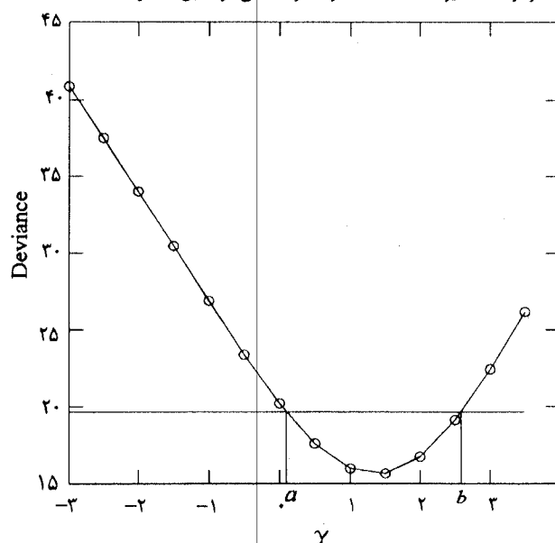
نمودار (۲) - مقادیر مشاهده شده انحراف درست‌نمایی در مقابل مقادیر مختلف \gamma
