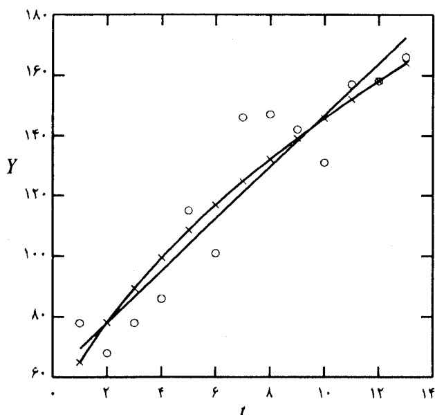
نمودار (۱) - مشاهدات (o) توان دوم خطی (x) و همانی خطی (خط مستقیم)
